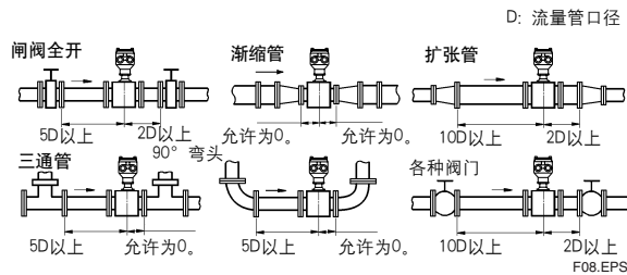
直管段长度
